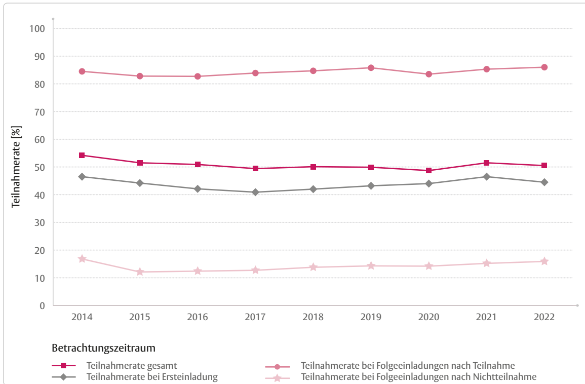
Abbildung 4: Teilnahme rate in Deutschland 2014–2022 nach Einladung s art
